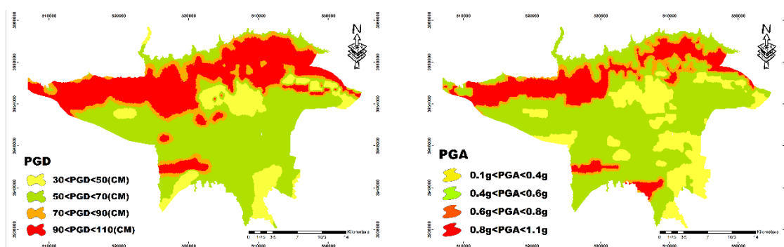
شکل ۲. نقشه PGA (بیشینه شتاب سطح زمین)
