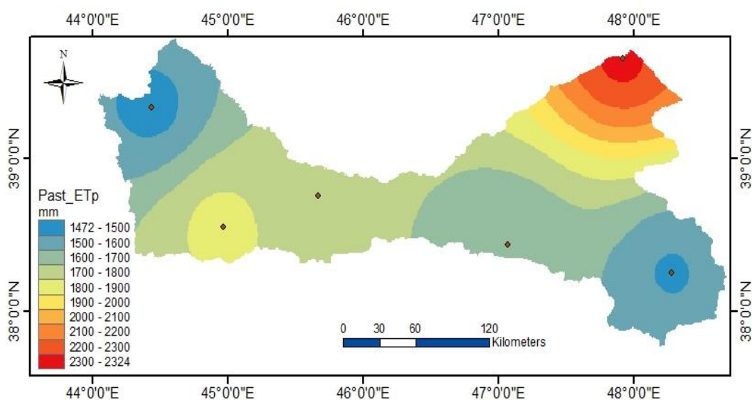
شکل ۴. پراکنش فضایی ET_p سالانه حوزه ارس در دوره پایه (۱۹۸۵-۲۰۰۵) بر مبنای داده‌های مدل GFDL
