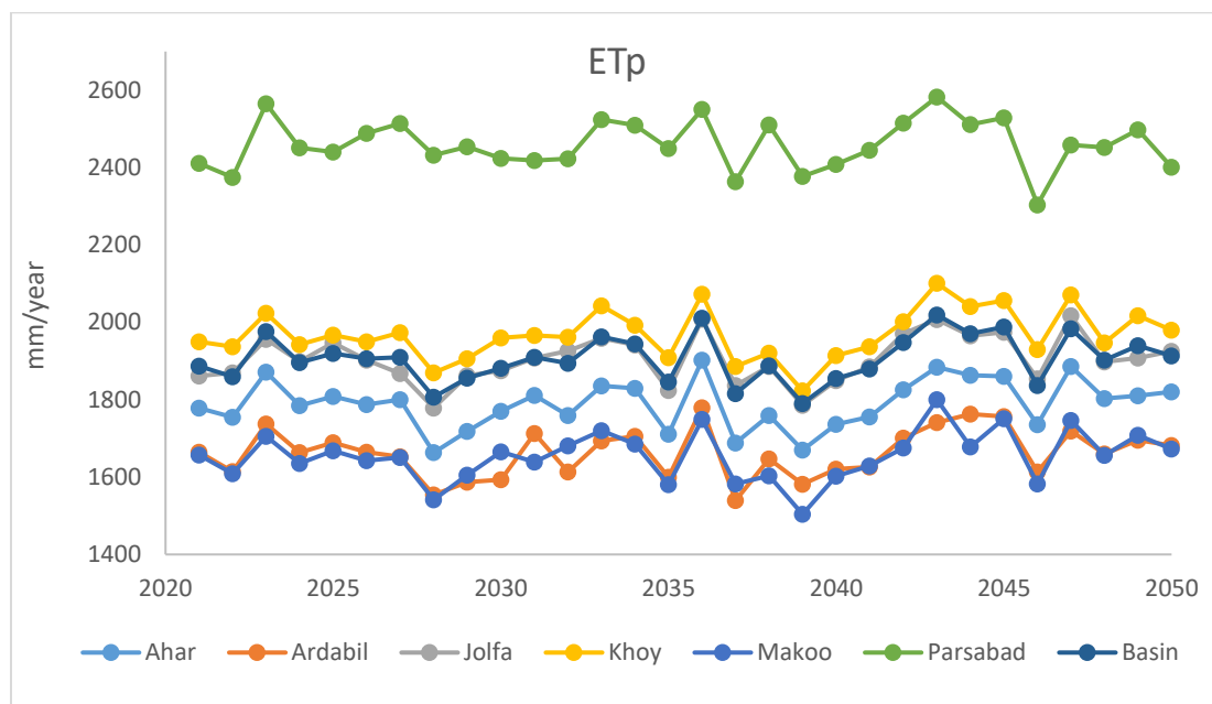
شکل ۳. ET_p برآوردی حوزه ارس برای دوره آینده (۲۰۲۱-۲۰۵۰) به روش هارگریوز-سامانی بر مبنای داده‌های مدل GFDL
