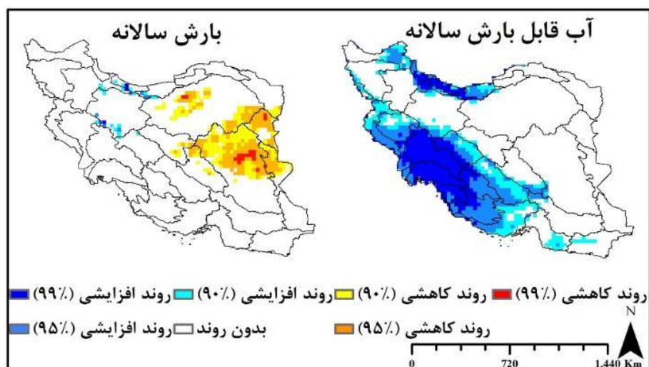
شکل ۱۰. روند تغییرات بارش و آب‌قابل‌بارش سالانه ایران (۱۹۷۹-۲۰۱۹)
