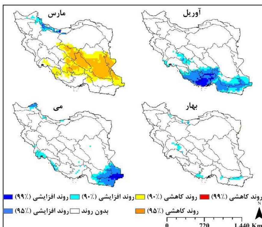
شکل ۶. روند تغییرات آب‌قابل‌بارش ماهانه (مارس، آوریل و می) و فصل بهار (۱۳۹۹-۱۳۹۷)
