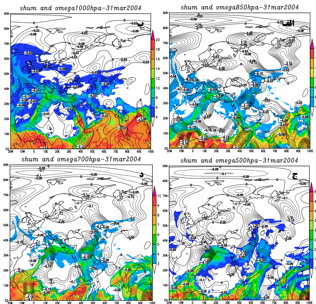
شکل ۱۲. نقشه های ترکیبی نم ویژه و امگای الگوی دوم در ترازهای ۱۰۰۰ تا ۵۰۰ هکتوپاسکال روز نماینده ۳۱ مارس ۲۰۰۴
