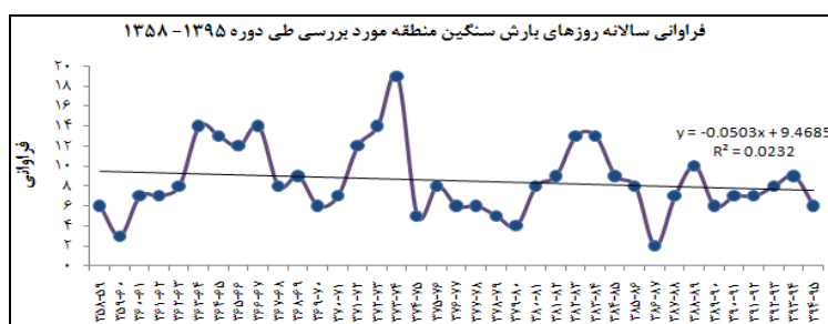
شکل ۴. روند فراوانی روزهای بارش سنگین منطقه مورد مطالعه طی دوره ۱۳۵۸-۱۳۹۵
