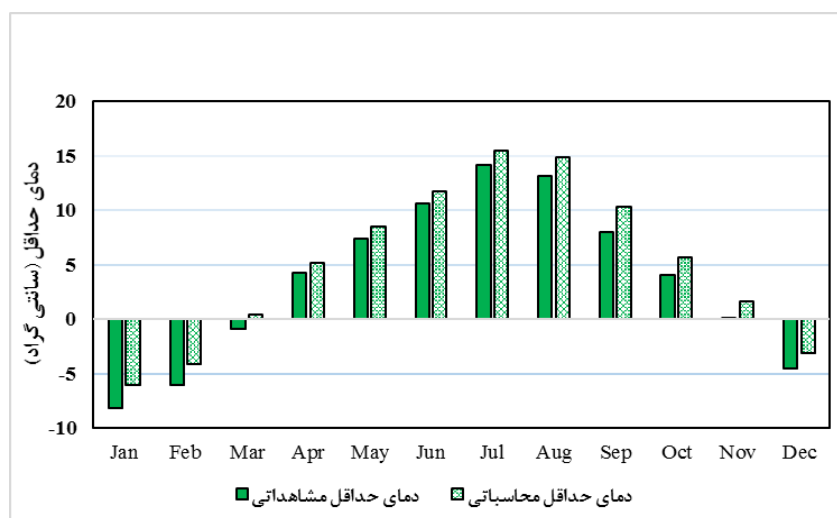
شکل ۹. مقایسه میانگین دمای حداقل ماهانه مشاهده‌ای دوره پایه با محاسباتی در دوره آبی در ایستگاه همدان.
