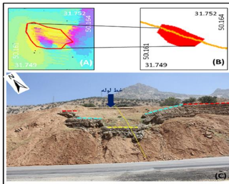
(A) انترفروگرم معرف زمین لغزش B موقعیت زمین لغزش ترسیمی نسبت به خط لوله C نمای شمال شرقی جنوبغربی از زمین لغزش حادث - خط زرد ممتد مسیر ترسیم پرفیل طولی ترسیم در قسمت B شکل ۱۲ - خطوط خط چین رنگی معرف اقدامات عمرات نا کارآمدی و بعضا تشدید کنند لغزش در مجاورت خط لوله از زمین لغزش مورد بررسی مطالعاتی و تداخل نگار مربوطه (A)
