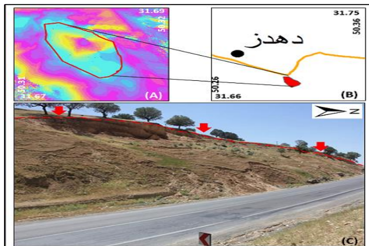
شکل ۹. عکس میدانی - نمونه‌ای از زمین لغزش حادث در مجاورت خط لوله در روستای دهدز (A) انترفروگرم معرف زمین لغزش B موقعیت زمین لغزش ترسیمی نسبت به خط لوله C نمای شرقی - غربی از زمین لغزش مورد بررسی - خطوط محل عبور تقریبی خط لوله را نشان می دهد.
