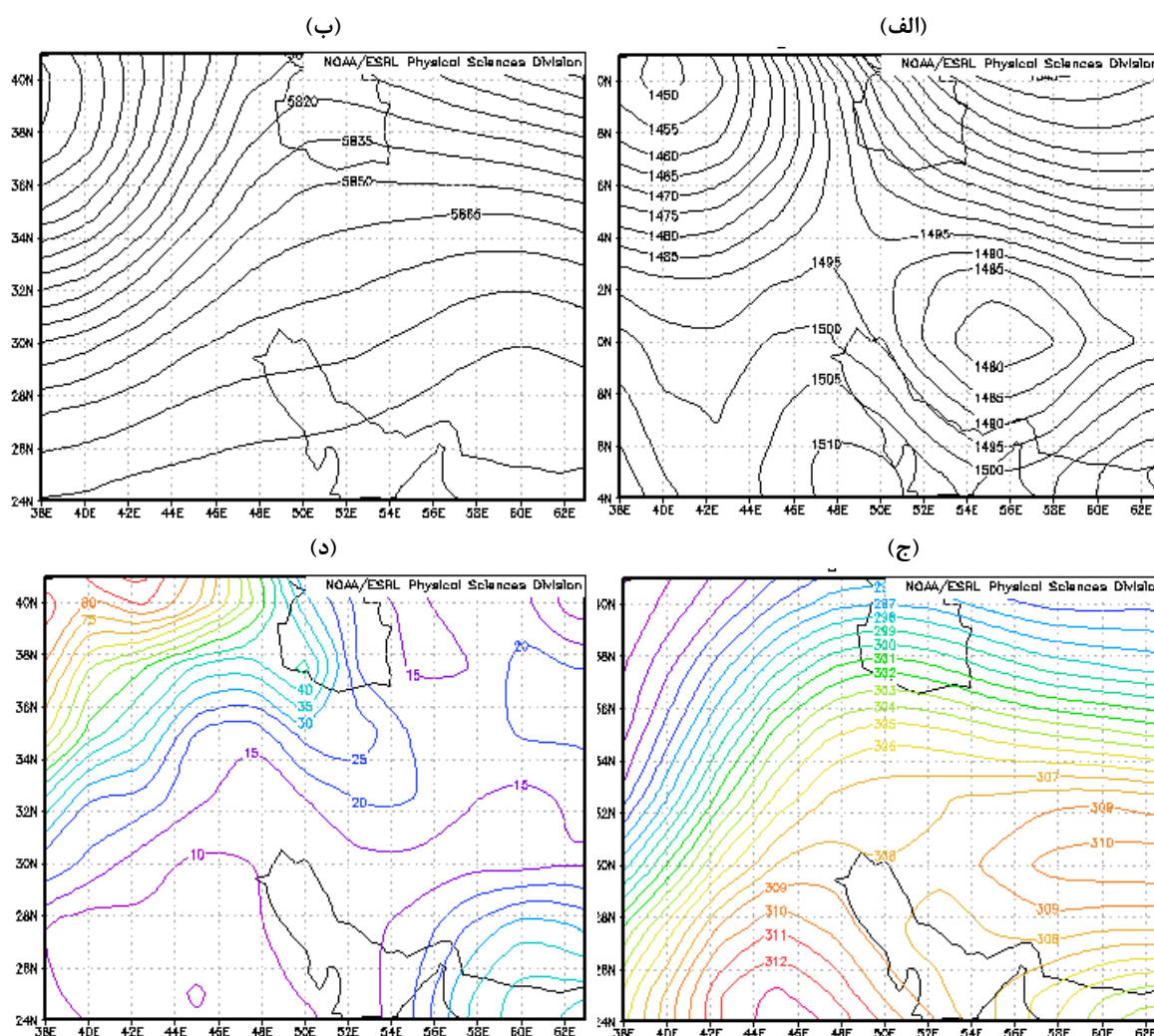
شکل ۷. مانند شکل ۴ ولی برای میانگین ساعت ۱۲ تا ۱۸ UTC روز ۲ ژوئن ۲۰۱۴.
