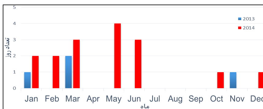
شکل ۳ مقایسه ماهانه رخداد با شرایط کمینه دید ۱۵۰۰ متر و تعداد روزها در سال‌های ۲۰۱۳ و ۲۰۱۴.
