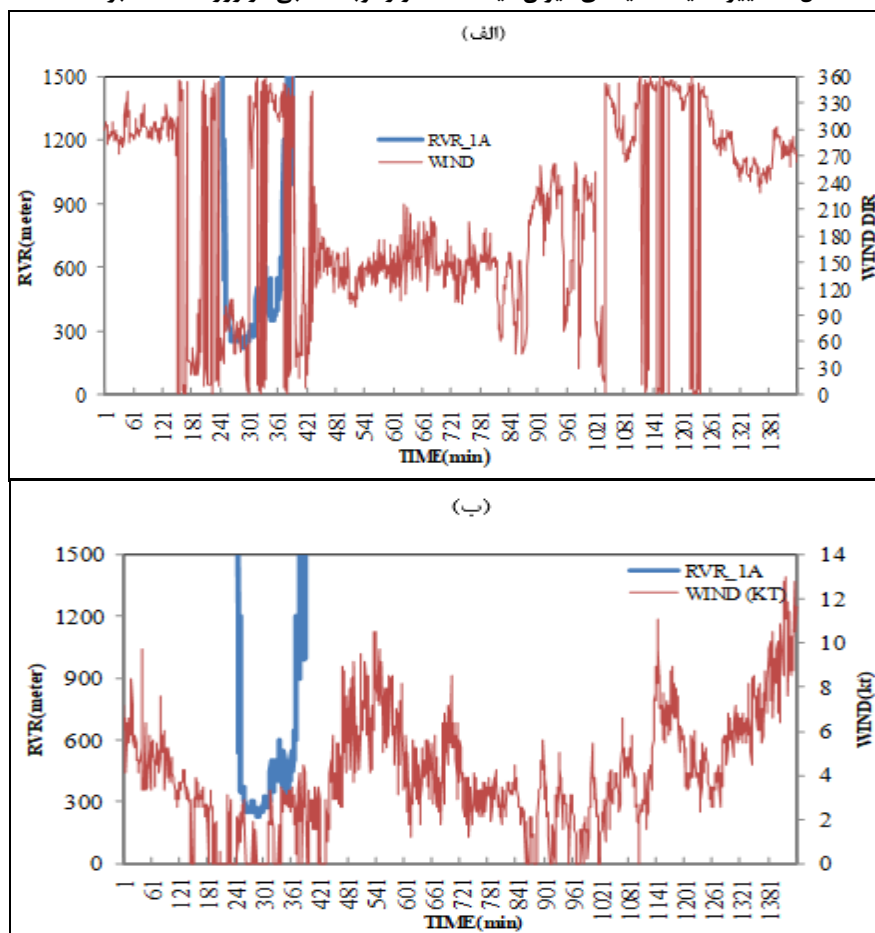
شکل ۶. تغییرات یک دقیقه‌ای (الف) دید RVR و جهت باد، (ب) دید RVR و تندی باد در روز ۲۳ دسامبر ۲۰۱۴.
