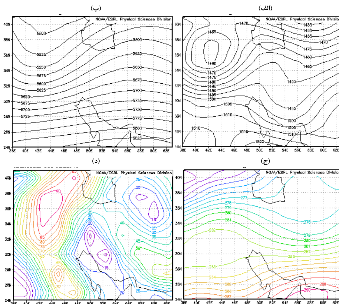
شکل ۴. نقشه‌های همدیدی ارتفاع ژئوپتانسیلی در سطوح (الف) ۸۵۰ و (ب) ۵۰۰ هکتوپاسکال، (ج) دما و (د) رطوبت نسبی (برحسب درصد) برای میانگین ساعت UTC ۰۶۰۰ تا ۰۰ روز ۲۳ دسامبر ۲۰۱۴.
