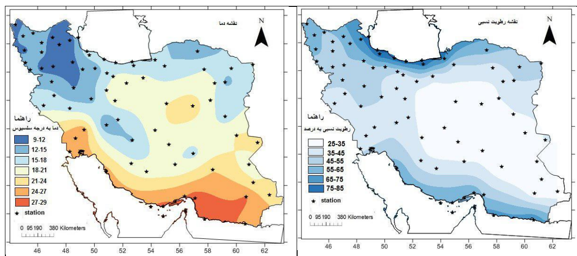
شکل ۲- نقشه توزیع فضایی میانگین دمای سالانه (سمت چپ) و میانگین رطوبت نسبی سالانه (سمت راست) ایران (۱۹۸۷-۲۰۱۶)
