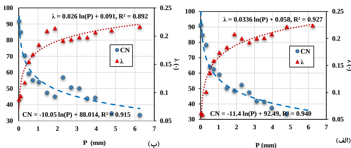
شکل ۵) رابطه بین مقادیر واسنجی شده (CN-P) و ( \lambda -P) در حوضه آبریز الف) پس قله و ب) مقصودبیک.
