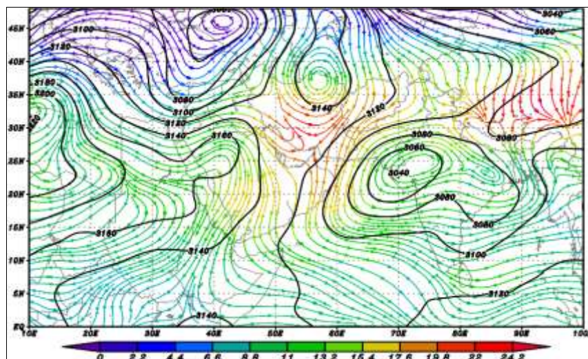
شکل ۱۷. نقشه ترکیبی ارتفاع ژئوپتانسیل و وزش دمای سطح ۷۰۰ هکتوپاسکال در موج گرمای شدید
