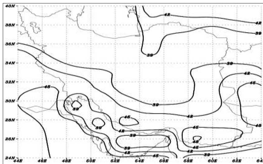
شکل ۱۴. دمای بیشینه دومتري سطح زمین در گرم ترین روز موج گرمایی ضعیف ۲۹ ژوئیه ۱۹۷۷
