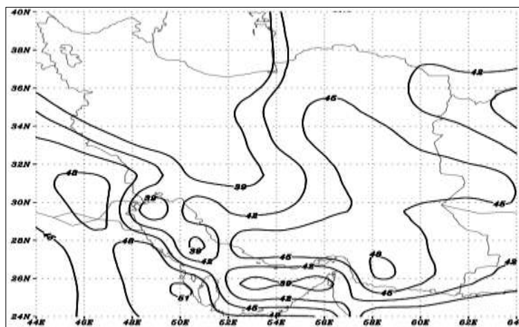
شکل ۱۹. دمای بیشینه دومتري سطح زمين در گرم ترين موج گرمایی ضعيف ۵ ژوئيه ۱۹۹۸
