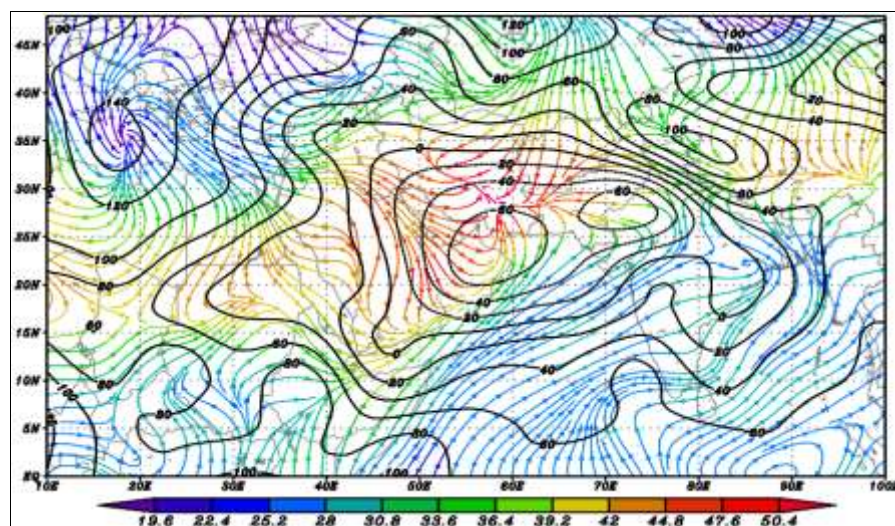
شکل ۱۸. نقشه ترکیبی ارتفاع ژئوپتانسیل و وزش دمای سطح ۱۰۰۰ هکتوپاسکال در موج گرمای شدید
