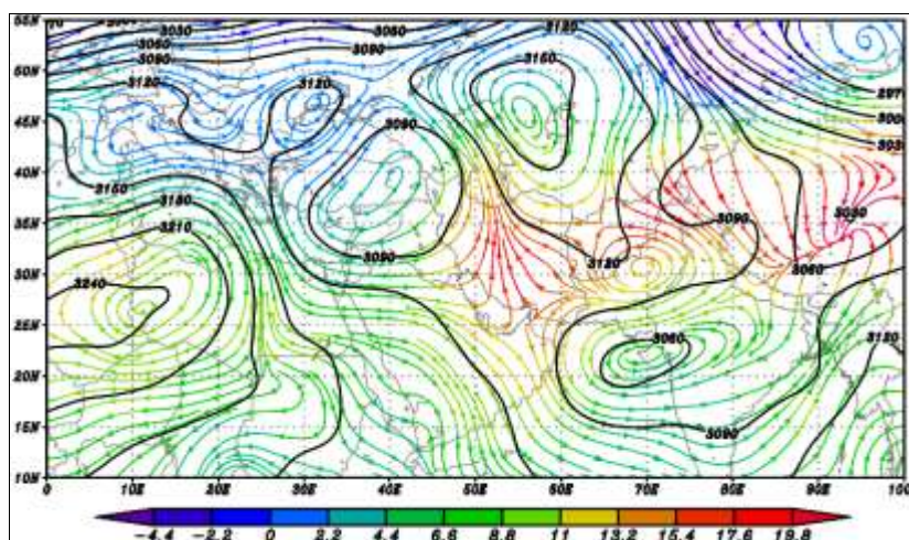
شکل ۷. نقشه ترکیبی ارتفاع ژئوپتانسیل و وزش دمایی تراز ۷۰۰ هکتوپاسکال در موج ضعیف
