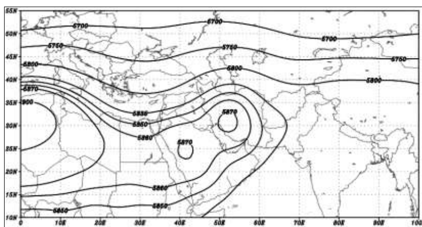
شکل ۷. نقشه بلند مدت ارتفاع ژئوپتانسیل سطح ۵۰۰ هکتوپاسکال در دوره سی ساله ۱۹۷۱-۲۰۰۰
