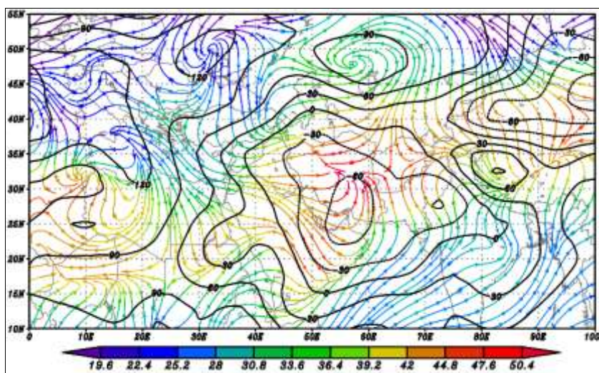
شکل ۸. نقشه ترکیبی ارتفاع ژئوپتانسیل و وزش دمایی تراز ۱۰۰۰ هکتوپاسکال در موج ضعیف
