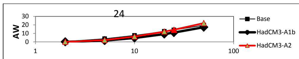
شکل ۱۳: شدت تجمعی خشکسالی به ترتیب از بالا به پایین برای تداوم زمانی ۳، ۱۲ و ۲۴ ماهه در دوره مشاهداتی، A۱B و A۲ و برای دوره برگشت ۲ تا ۵۰ سال برای مناطق جنوبی ایران
