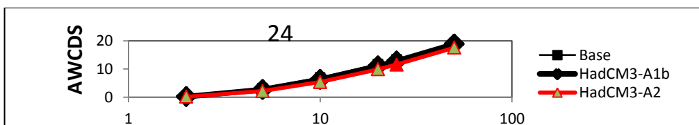
شکل ۱۲: شدت تجمعی خشکسالی به ترتیب از بالا به پایین برای تداوم زمانی ۳، ۱۲ و ۲۴ ماهه در دوره مشاهداتی، A۱B و A۲ و برای دوره برگشت ۲ تا ۵۰ سال برای مناطق مرکزی ایران
