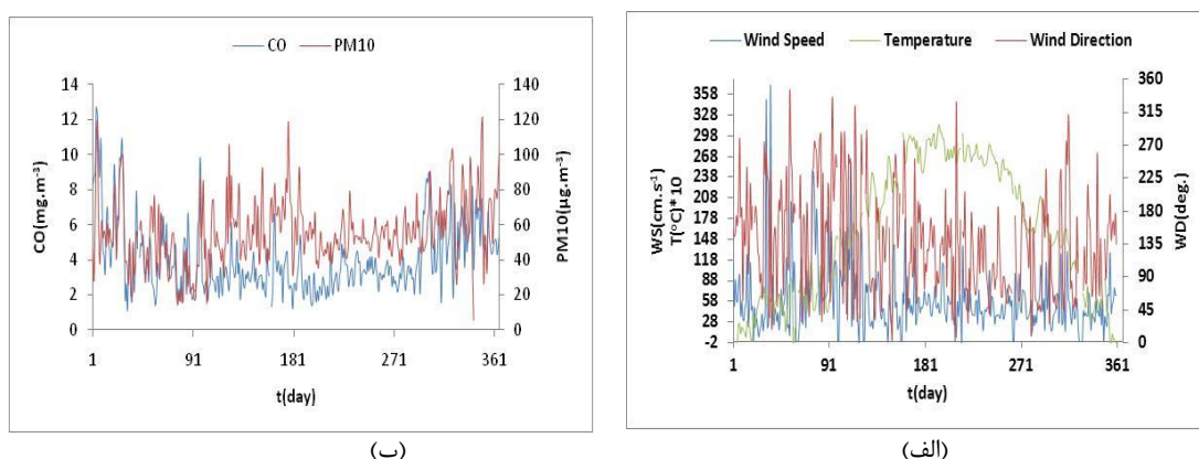
شکل ۷. نمودار چرخه‌ی سالانه تغییرات میانگین شبانه‌روزی، (الف) تندى (برحسب سانتی‌متر بر ثانیه) و جهت باد و دماى هوا و (ب) CO و PM 10 در سال ۲۰۰۷.
