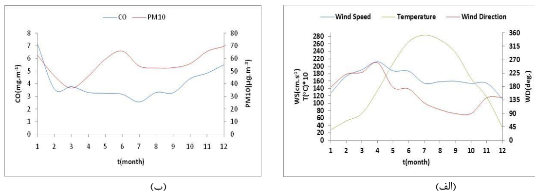
شکل ۲. چرخه‌ی سالانه، الف) تندی و جهت باد و دما و ب) CO و PM 10 بر اساس میانگین‌های ماهانه در سال ۲۰۰۷.
