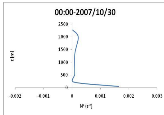
شکل ۳. نیمرخ قائم توان دوم بسامد شناوری، الف) در تاریخ ۲۷/۱/۲۰۰۷، ساعت ۰۰:۰۰ UTC (سمت راست)، ساعت ۱۲:۰۰ UTC (سمت چپ)، ب) در تاریخ ۱۲/۶/۲۰۰۷، ساعت ۰۰:۰۰ UTC (پ) در تاریخ ۶/۷/۲۰۰۷، ساعت ۰۰:۰۰ UTC (ت) در تاریخ ۳۰/۱۰/۲۰۰۷، ساعت ۰۰:۰۰ UTC.
