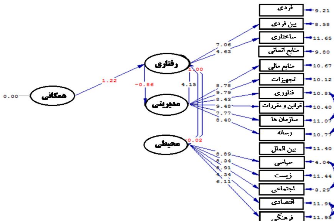
شکل ۳. خروجی نرم افزار از مقادیر استاندارد در تحلیل مسیر
