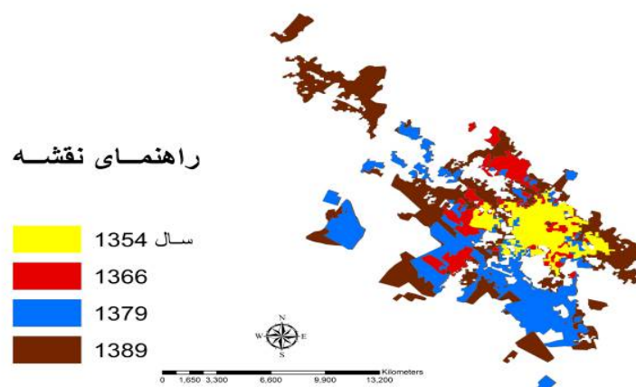
شکل (۴) رشد و گسترش افقی شهر یزد در دوره های مختلف (ترسیم بر اساس رقومی کردن تصاویر ماهواره ای از سنجنده ETM+ دوره های مختلف مورد بررسی با انجام تصحیحات رادیومتریکی).
