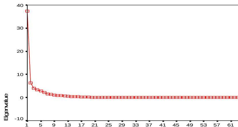
شکل (۳) سهم هر مولفه EOF در برآورد واریانس کل EOFS
