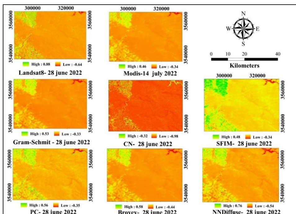
شکل (۷). شاخص پوشش گیاهی (NDVI) الگوریتم‌های تلفیق مورد بررسی و تصویر ماهواره‌ای لندست-۸ و مادیس
