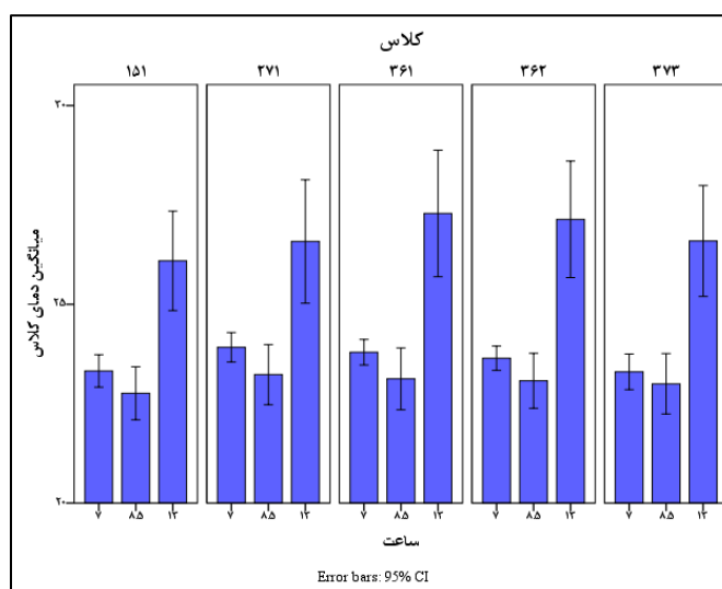
شکل (۴). میانگین دمای کلاس در ساعت‌های منتخب
