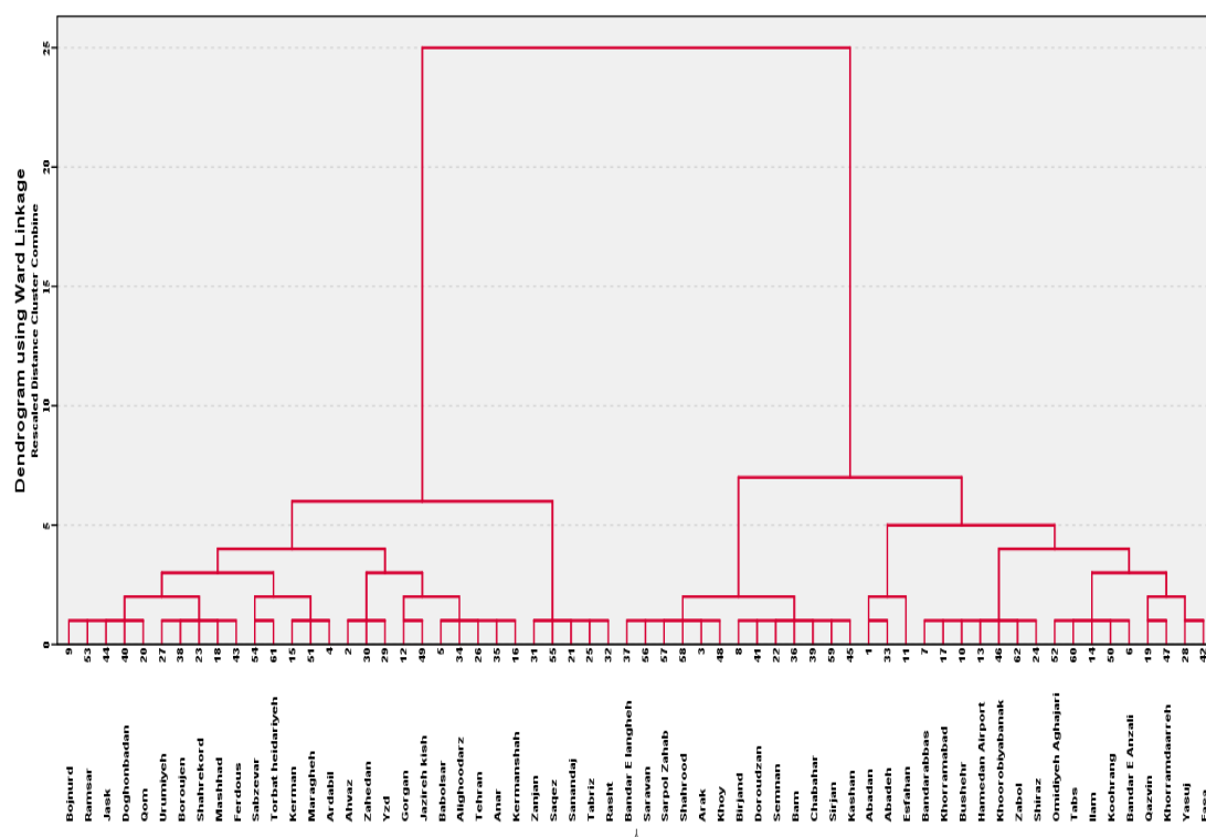
شکل (۴). درخت خوشه‌بندی روند تغییرات بارش شاخص‌های شدت بارش‌های یک تا شش روزه ایران
