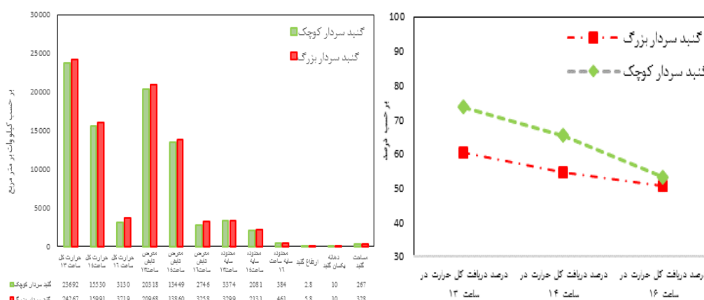
شکل (۸). نمودار از سمت چپ مربوط به میزان دریافت حرارت در معرض تابش، در محدوده‌ی سایه و حرارت کل گنبد آب‌انبارهای دهانه ثابت شهر قزوین در سردترین روز سال در ساعات ۱۳، ۱۴، ۱۶. نمودار از راست درصد میزان دریافت تابش خورشید بر سطوح گنبدهای با دهانه ثابت قزوین در ساعات ۱۴، ۱۶، ۱۸. منبع: نگارندگان.
