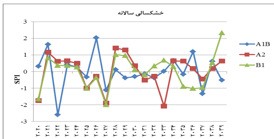
شکل (۸). خشکسالی سالانه تحت سه سناریوی A1B، A2 و B1 (۲۰۲۰-۲۰۳۹).
