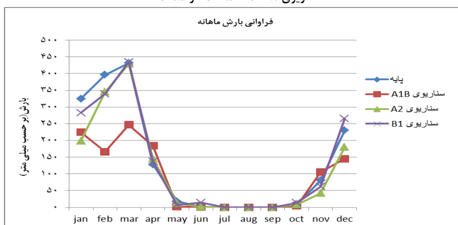
شکل (۴). مقایسه فراوانی بارش ماهانه در دوره پایه (۱۹۸۶-۲۰۱۵) و دوره آینده (۱۰۳۹-۲۰۲۰) تحت سه سناریوی A1B، A2 و B1.
