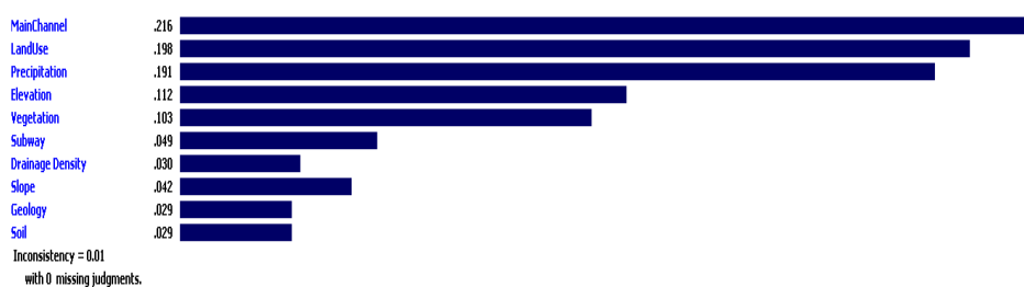
شکل (۳). وزن‌های بدست آمده برای معیارها و میزان ضریب ناسازگاری (منبع: نگارندگان)
