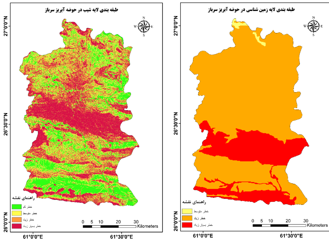
شکل (۵). طبقه‌بندی لایه زمین‌شناسی حوضه آبریز سرپاز بر حسب پتانسیل سیل‌خیزی (منبع: نگارندگان)
