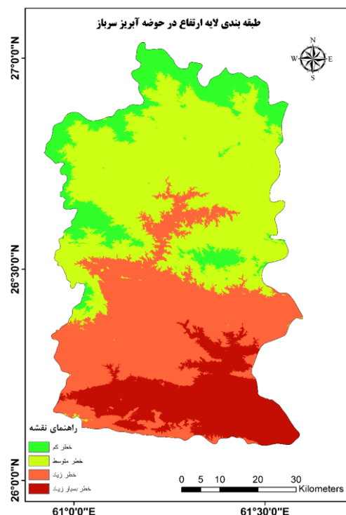
شکل (۴). طبقه‌بندی لایه ارتفاعی حوضه آبریز سرباز بر حسب پتانسیل سیل‌خیزی (منبع: نگارندگان)
