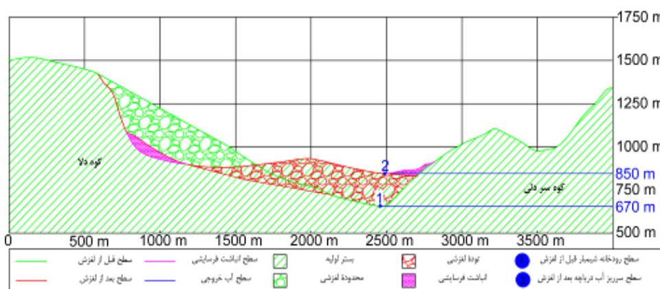
شکل (۸). نیمرخ عرضی سطح و توده لغزشی دلا
