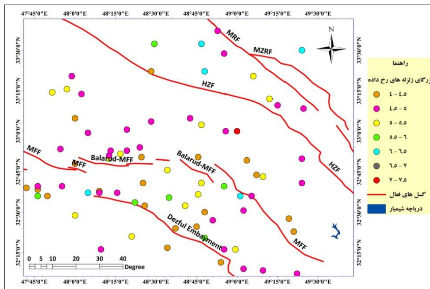
شکل (۶). گسل های فعال و زلزله های با بزرگای بیشتر از ۴ ریشتر در محدوده دریاچه شیمبار و اطراف آن (حسامی و جماله، ۲۰۰۶، زارع و همکاران، ۲۰۱۴).
