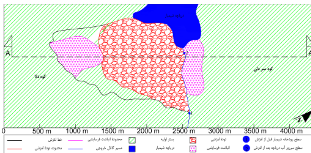
شکل (۷). یلان، سطح و توده لغزشی، دلا
