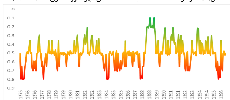
شکل (۹). نمودار SEPI ۶ ماهه ایستگاه پارس آباد مغان (دوره آماری ۱۹۹۶-۲۰۱۶)
