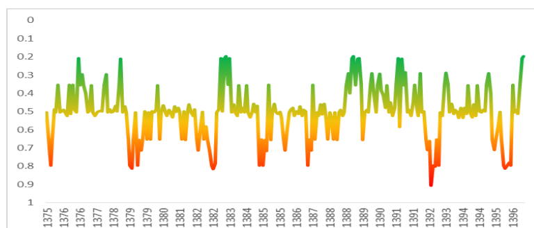
شکل (۸). نمودار SEPI ۶ ماهه ایستگاه مشکین شهر (دوره آماری ۱۹۹۶-۲۰۱۶)
