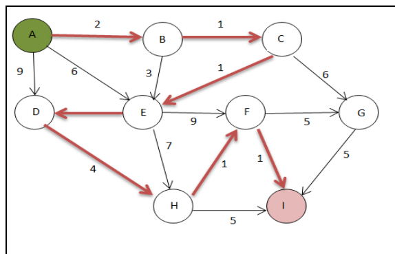
شکل (۱). نحوه عملکرد الگوریتم Dijkstra [Saberian and Hamrah, 1388].
