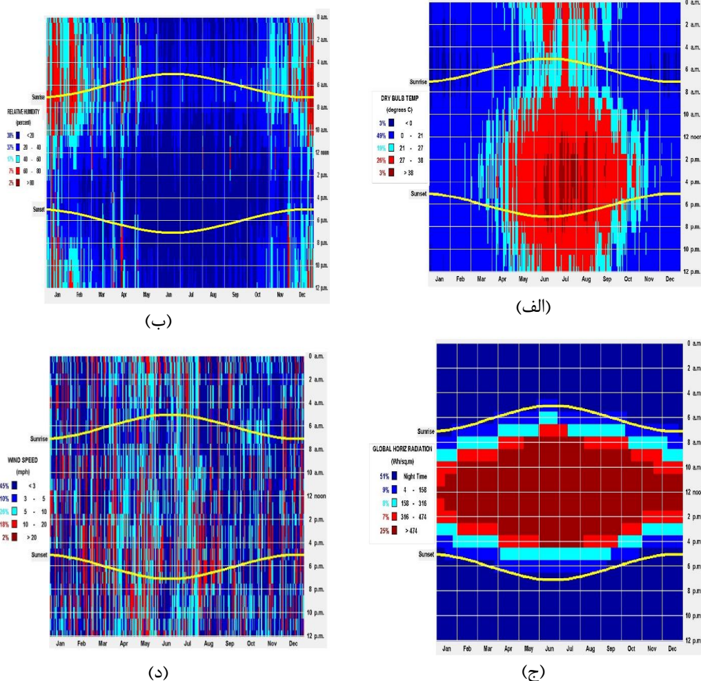
شکل (۱). بررسی زمانی شرایط آسایش حرارتی قبل و بعد از طلوع آفتاب در یزد (الف تا د) (منبع: نگارندگان، ۱۳۹۷)
