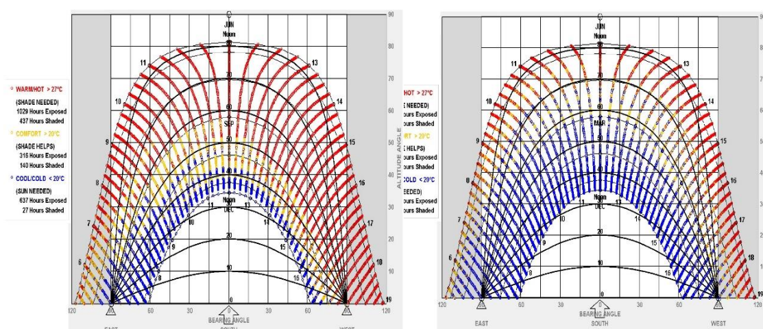
شکل (۲). شاخص عمودی خورشید دوره (زمستان-بهار) (منبع: نگارندگان، ۱۳۹۷) شکل (۳). شاخص عمودی خورشید دوره (تابستان-پاییز) (منبع: نگارندگان، ۱۳۹۷)
