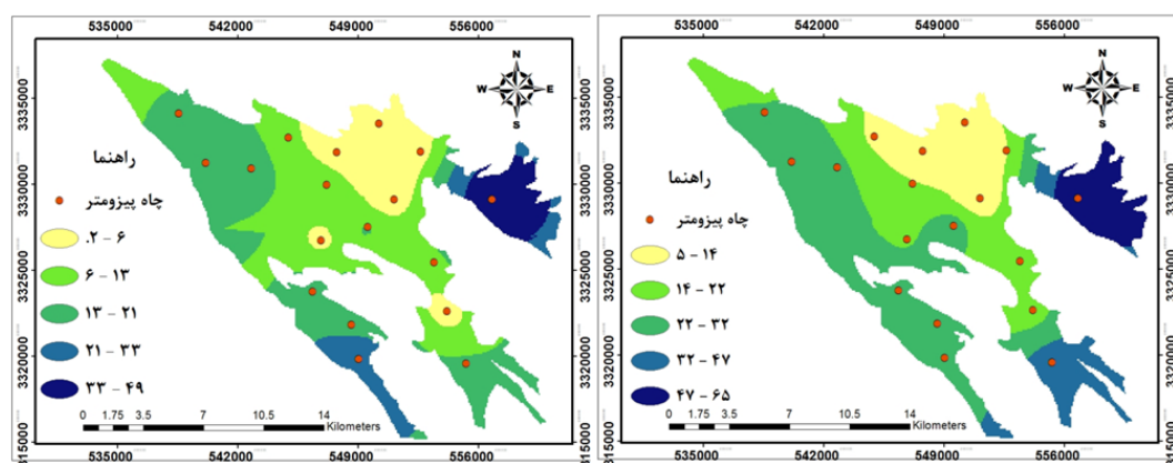
شکل (۶). الف: نقشه هم‌عمق آب زیرزمینی در سال ۱۳۸۸ ب: نقشه هم‌عمق آب زیرزمینی در سال ۱۳۸۲
