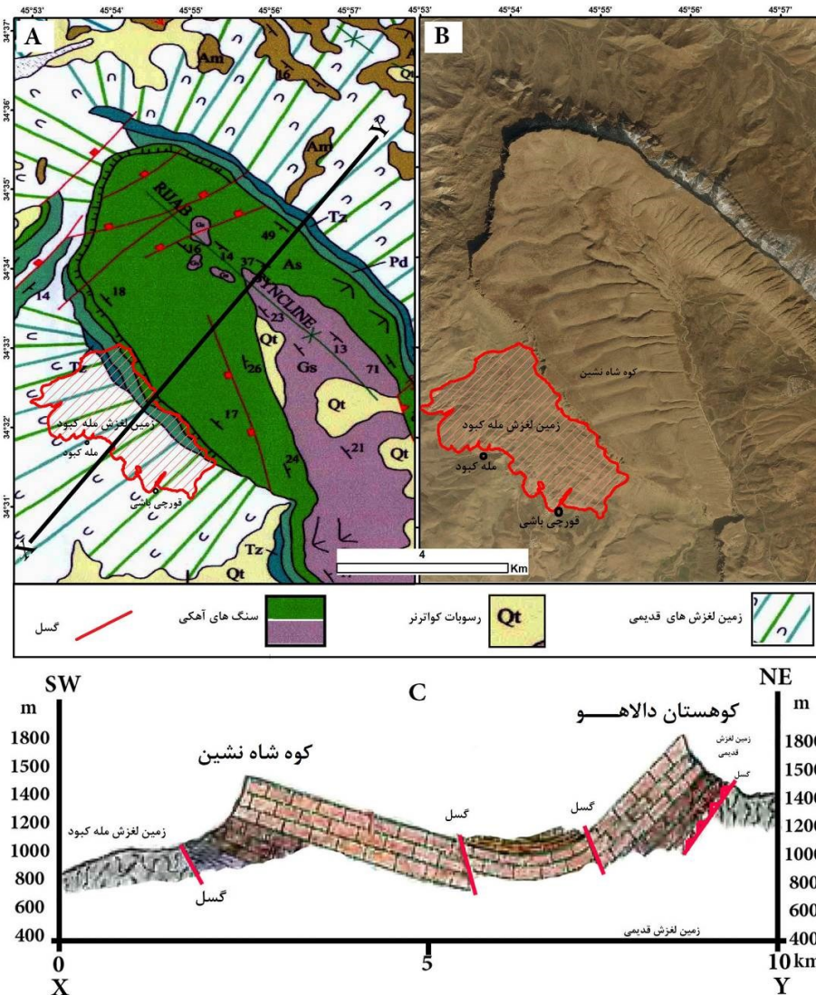
شکل (۲). موقعیت زمین ساختی - مورفوتکتونیکی (A) و مورفولوژیکی (B) زمین لغزش مله کبود (C)
