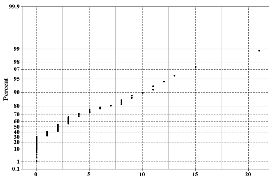
شکل (۲). توزیع احتمال مقادیر فرین بیشینه برای فراوانی وقوع توفان‌های گرد و خاک ایستگاه خرم‌آباد در ماه مه
