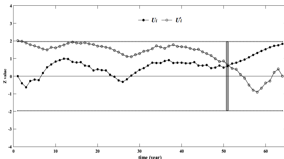
شکل (۱۶). نمودار من‌کندال برای آشکارسازی روند تغییرات سالانه فراوانی وقوع توفان‌های گرد و غباری خرم‌آباد
