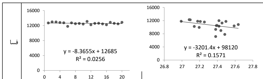
شکل (۸). ارتباط عملکرد دانه ذرت با دمای بیشینه در شهرستان‌های منتخب در دو دوره آینده (اول ۲۰۱۱-۳۰ و دوم ۲۰۴۶-۶۵).
