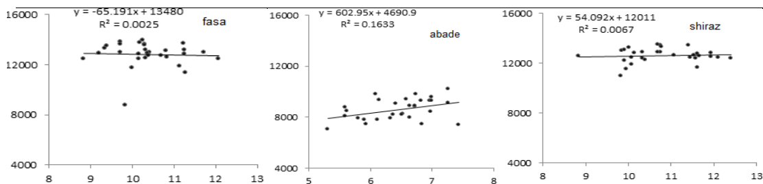
شکل (۳). ارتباط بین عملکرد دانه ذرت و دمای کمینه دوره پایه (۱۹۷۸-۲۰۱۶) در منطقه مورد بررسی
