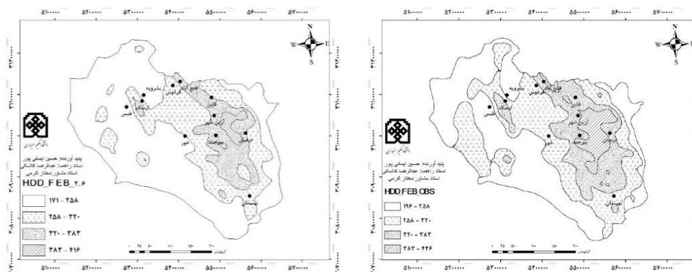
شکل (۲۲). پراکنش مکانی نیازهای گرمایشی ماه بهمن در شکل (۲۳). پراکنش مکانی نیازهای گرمایشی ماه بهمن در دوره مشاهده ای (۱۹۹۰-۲۰۱۵) دوره آینده (۲۰۱۶-۴۱)، سناریو RCP_2.6
