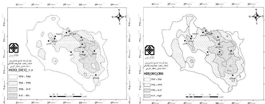
شکل (۱۴). پراکنش مکانی نیازهای گرمایشی آذر در دوره مشاهده ای (۱۹۹۰-۲۰۱۵) شکل (۱۵). پراکنش مکانی نیازهای گرمایشی آذر در دوره
