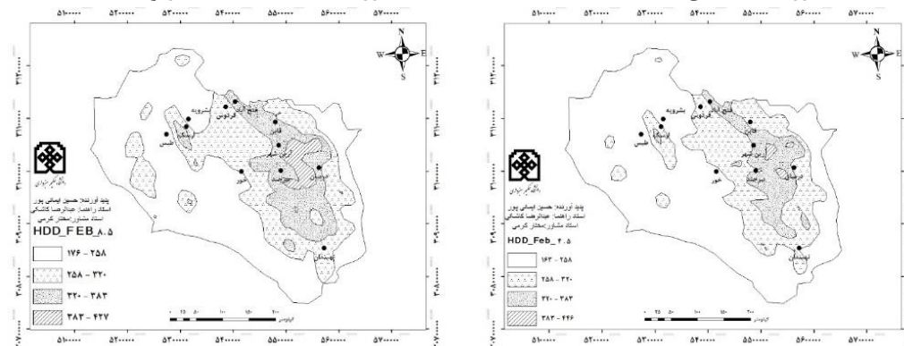
شکل (۲۴). پراکنش مکانی نیازهای گرمایشی بهمن در شکل (۲۵). پراکنش مکانی نیازهای گرمایشی بهمن دوره آینده (۲۰۱۶-۴۱)، سناریو RCP_4.5 دوره آینده (۲۰۱۶-۴۱)، سناریو RCP_8.5
