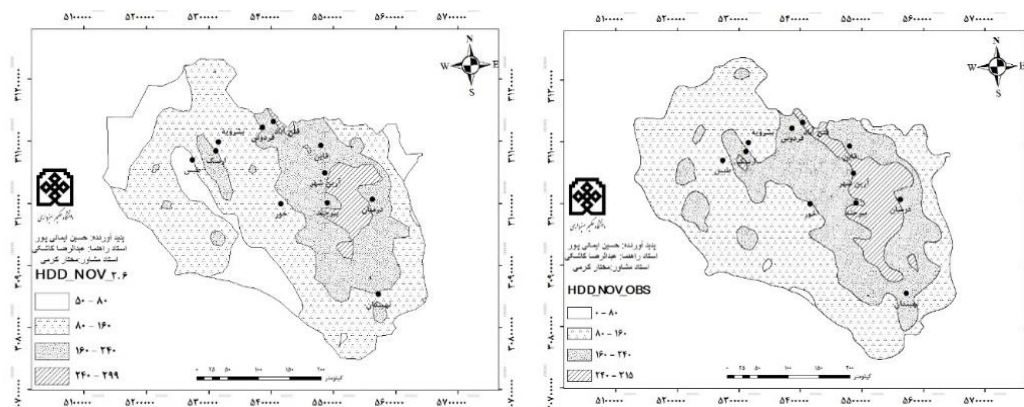
شکل (۱۰). پراکنش مکانی نیازهای گرمایشی ماه آبان در دوره مشاهده ای (۱۹۹۰-۲۰۱۵)
