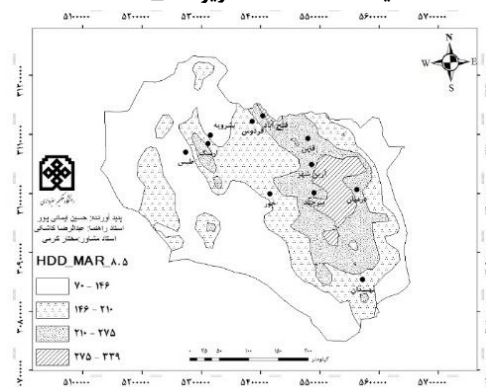
شکل (۲۹). پراکنش مکانی نیازهای گرمایشی اسفند، دوره آینده (۲۰۱۶-۴۱) سناریو RCP_8.5
