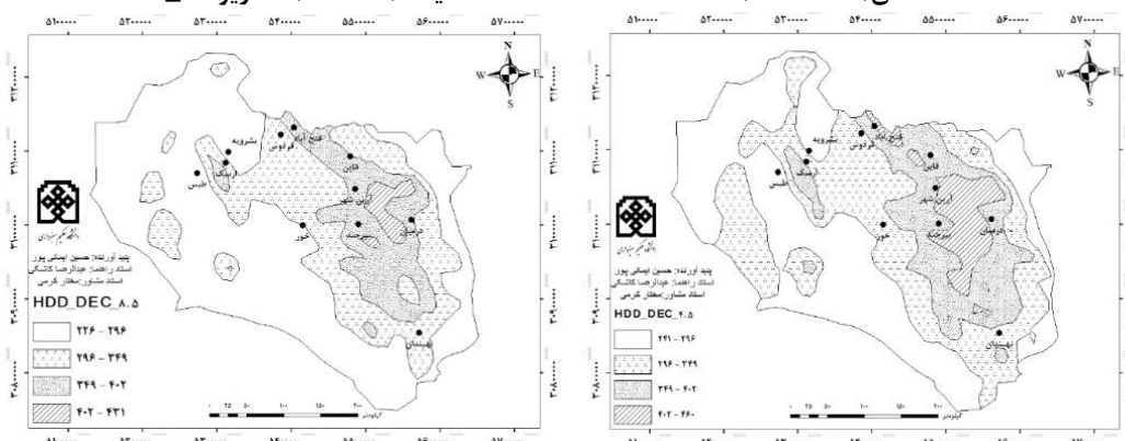
شکل (۱۷). پراکنش مکانی نیازهای گرمایشی آذر در دوره
