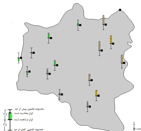
شکل (۴). مقایسه بین سطح آب زیرزمینی محاسبه شده و مشاهده شده.
