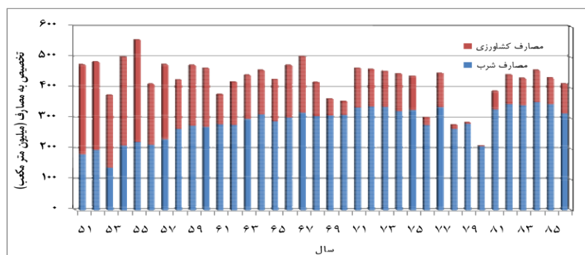
شکل (۱۳). حجم آب تنظیم یافته سد کرج جهت مصارف کشاورزی و شرب
