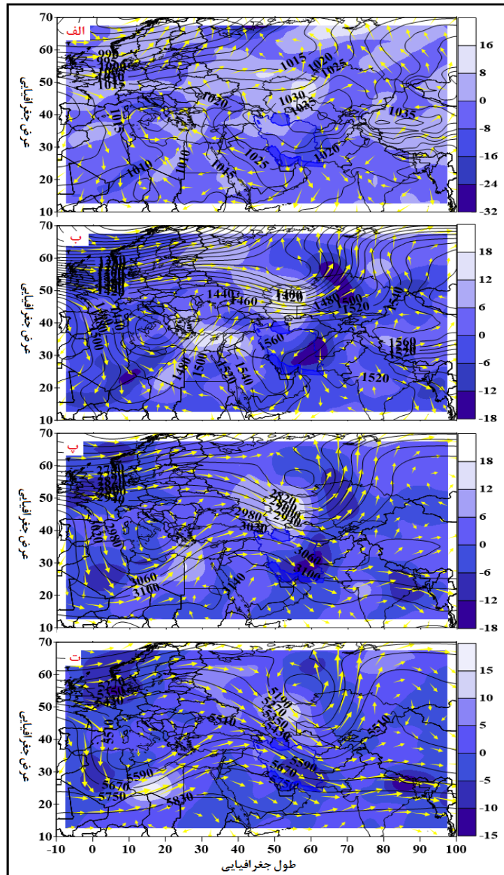
شکل (۳): نقشه الف: فشار تراز ۱۰۰۰ هکتوپاسکال، فرارفت دمای برحسب سانتیگراد، مؤلفه جریان باد برحسب متربرثانیه. نقشه ب: ارتفاع تراز ۸۵۰ هکتوپاسکال برحسب ژئوپتانسیل متر، فرارفت دمای برحسب سانتیگراد، مؤلفه جریان باد برحسب متربرثانیه. نقشه پ: ارتفاع تراز ۷۰۰ هکتوپاسکال برحسب ژئوپتانسیل متر، فرارفت دمای برحسب سانتیگراد، مؤلفه جریان باد برحسب متربرثانیه. نقشه ت: ارتفاع تراز ۵۰۰ هکتوپاسکال برحسب ژئوپتانسیل متر، فرارفت دمای برحسب سانتیگراد، مؤلفه جریان باد برحسب متربرثانیه.
