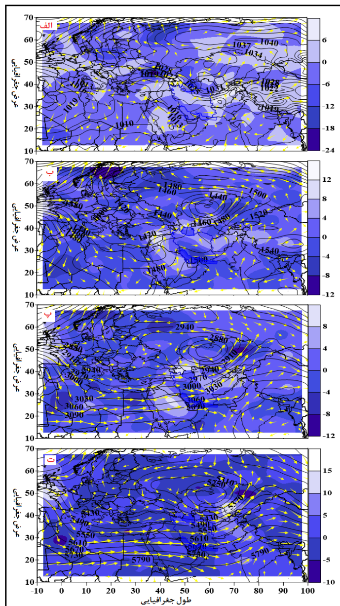
شکل (۲): نقشه الف: فشار تراز ۱۰۰۰ هکتوپاسکال، فرارفت دمای برحسب سانتیگراد، مؤلفه جریان باد برحسب متربرثانیه. نقشه ب: ارتفاع تراز ۸۵۰ هکتوپاسکال برحسب ژئوپتانسیل متر، فرارفت دمای برحسب سانتیگراد، مؤلفه جریان باد برحسب متربرثانیه. نقشه پ: ارتفاع تراز ۷۰۰ هکتوپاسکال برحسب ژئوپتانسیل متر، فرارفت دمای برحسب سانتیگراد، مؤلفه جریان باد برحسب متربرثانیه. نقشه د: ارتفاع تراز ۵۰۰ هکتوپاسکال برحسب ژئوپتانسیل متر، فرارفت دمای برحسب سانتیگراد، مؤلفه جریان باد برحسب متربرثانیه.
