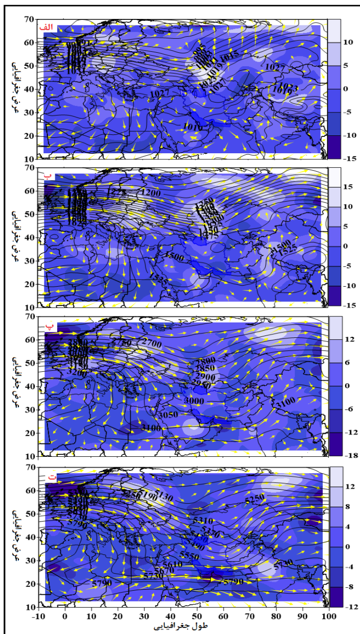
شکل (۴): نقشه الف: فشار تراز ۱۰۰۰ هکتوپاسکال، فرارفت دمای برحسب سانتیگراد، مؤلفه جریان باد برحسب متربرثانیه. نقشه ب: ارتفاع تراز ۸۵۰ هکتوپاسکال برحسب ژئوپتانسیل متر، فرارفت دمای برحسب سانتیگراد، مؤلفه جریان باد برحسب متربرثانیه. نقشه پ: ارتفاع تراز ۷۰۰ هکتوپاسکال برحسب ژئوپتانسیل متر، فرارفت دمای برحسب سانتیگراد، مؤلفه جریان باد برحسب متربرثانیه. نقشه ت: ارتفاع تراز ۵۰۰ هکتوپاسکال برحسب ژئوپتانسیل متر، فرارفت دمای برحسب سانتیگراد، مؤلفه جریان باد برحسب متربرثانیه.
