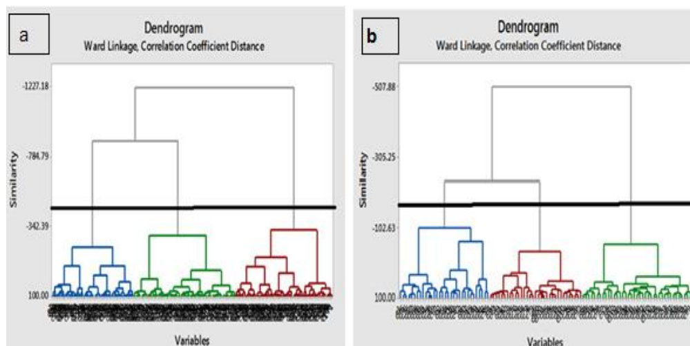
شکل (۲). نمودار درختی حاصل از تحلیل خوشه ای بر روی مقادیر روزهای بارش فراگیر در طول دوره آماری. داده های افرودیت (a) داده های ایستگاهی (b)
