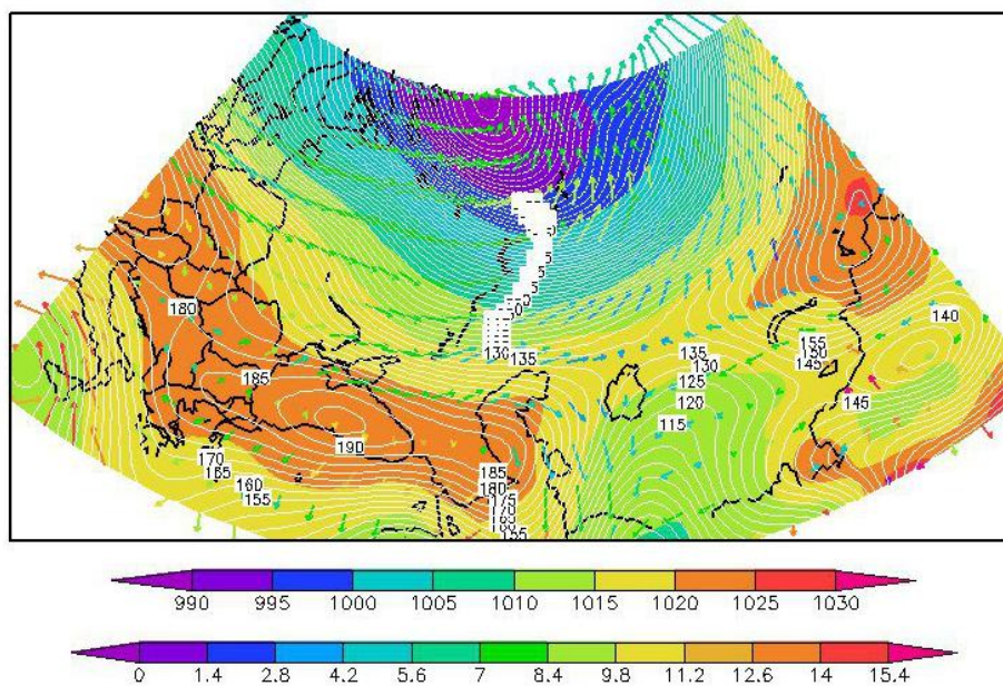
شکل (۱۰). نماینده الگوی پرفشار مهاجر در سطح ۱۰۰۰ هکتوپاسکال
