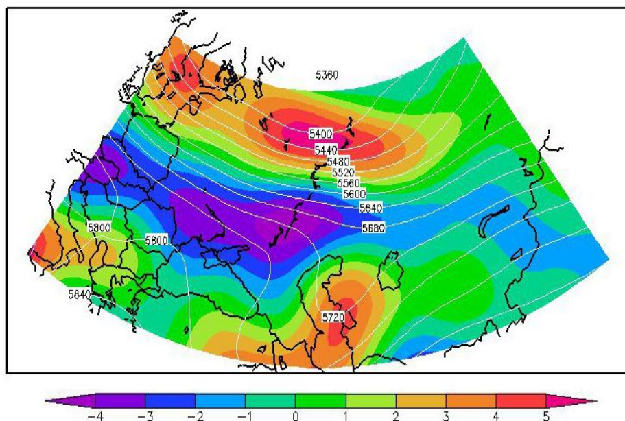
شکل (۱۱). نماینده الگوی پرفشار مهاجر در سطح ۵۰۰ هکتوپاسکال
