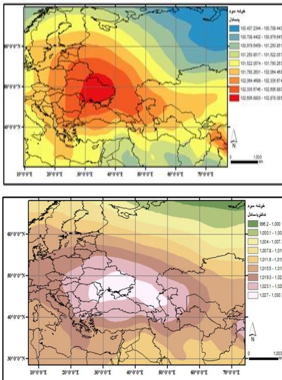
شکل (۵). (الف) مقایسه نقشه میانگین خوشه الگوی پرفشارمهاجر مربوط به داده های افرویت و (ب) داده های ایستگاهی
