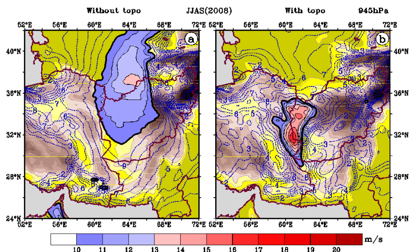
شکل (۱۲). شدت باد در شرایط با توپوگرافی (سمت راست) و بدون توپوگرافی (سمت چپ) شرق فلات ایران در تراز بیشینه سرعت باد (۹۴۵ ه.پ.). پربند سیاه پررنگ نشان‌دهنده سرعت باد ۱۰ متر بر ثانیه است.
