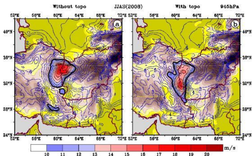
شکل (۵). شدت باد در شرایط با توپوگرافی (سمت راست) و بدون توپوگرافی خراسان جنوبی (سمت چپ) در تراز بیشینه سرعت باد (۹۴۵ ه.پ.). پررنگ سیاه پررنگ نشان دهنده سرعت باد ۱۰ متر بر ثانیه است.
