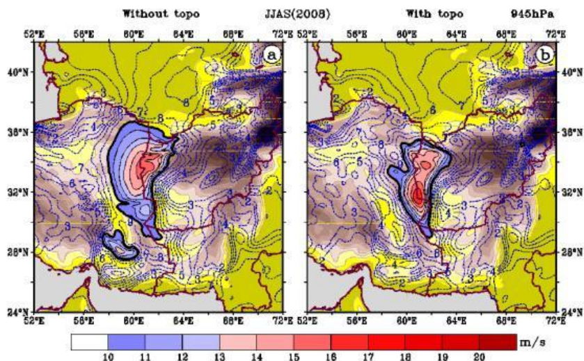
شکل (۹). شدت باد در شرایط با توپوگرافی (راست) و بدون توپوگرافی خراسان شمالی، رضوی و جنوبی (چپ) در تراز بیشینه سرعت باد (۹۴۵ ه.پ.). پربند سیاه پررنگ نشان‌دهنده سرعت باد ۱۰ متر بر ثانیه است.
