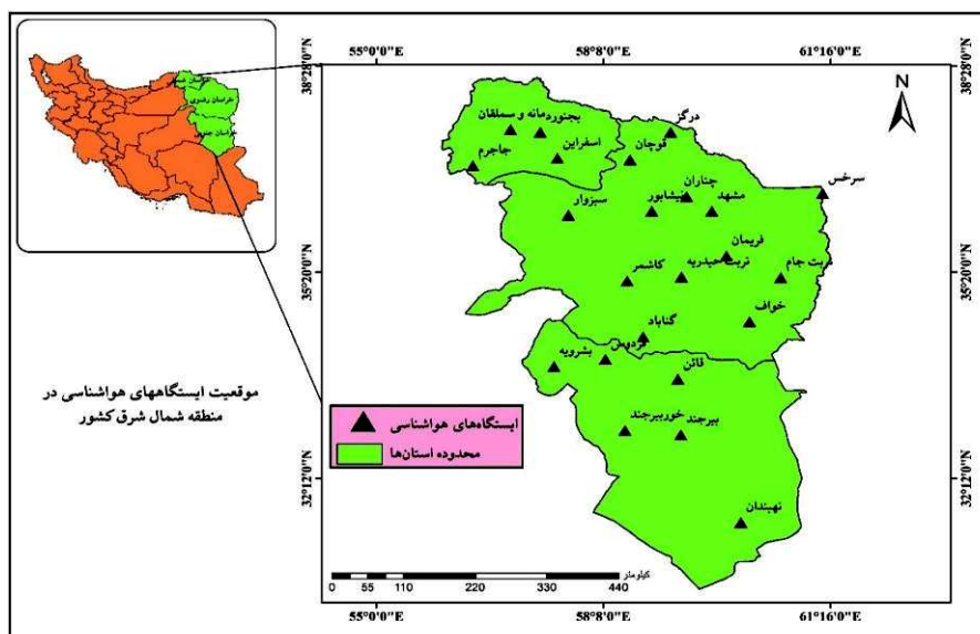
شکل (۳). نقشه‌ی موقع جغرافیایی منطقه‌ی مورد مطالعه و ایستگاه‌های سینو تیک منتخب
