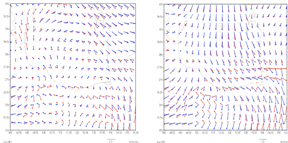
شکل (۹). نقشه بردار باد سطح زمین در ساعت ۱۲ GMT روز ۶ جولای ۲۰۰۲، شرایط مرجع (خطوط قرمز) و شرایط حاصل از حذف توپوگرافی (خطوط آبی)
