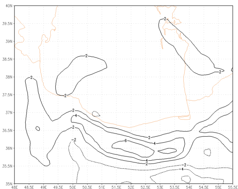
شکل (۴). تفاوت ماهانه دما سطح زمین به درجه سانتی گراد حاصل از تفاضل گیری بین شرایط حذف توپوگرافی و شرایط مرجع در ساعت GMT+۲
