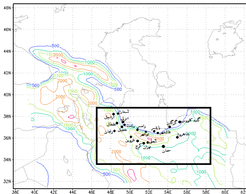
شکل (۲). محدوده مورد مطالعه (داخل کادر)، شرایط توپوگرافی مرجع و محدوده شبیه سازی شده
