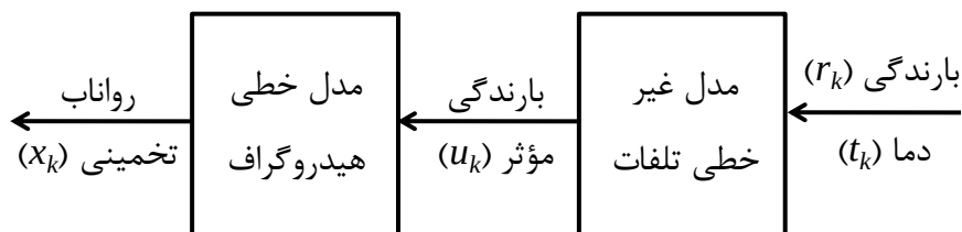
شکل (۳) چگونگی شبیه‌سازی بارش - رواناب در مدل IHACRES
