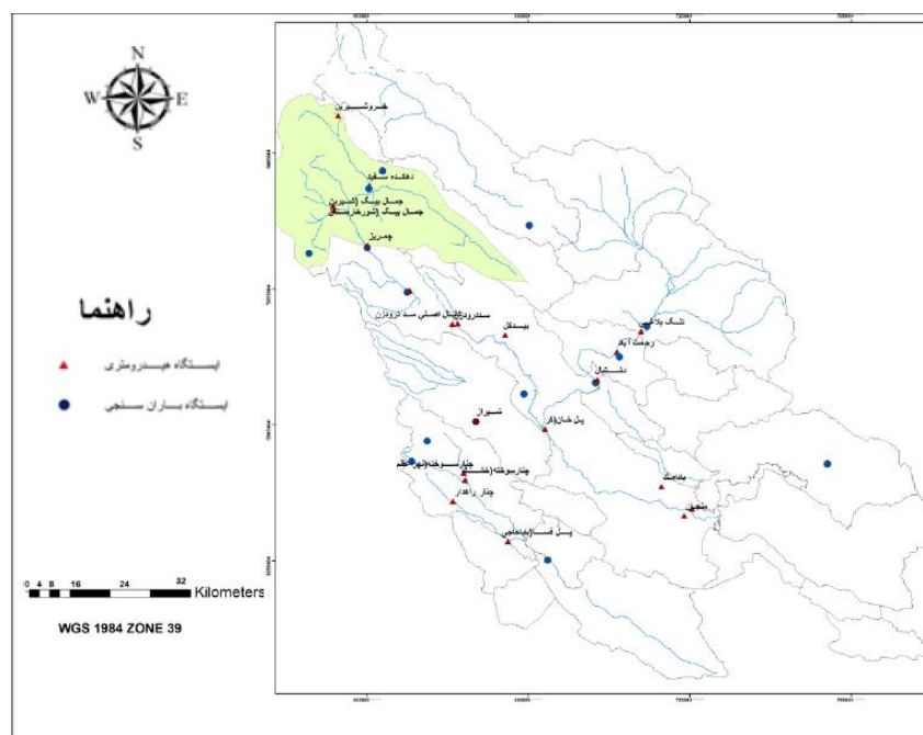
شکل (۲) موقعیت حوزه رودخانه کر و جانیابی ایستگاه‌های هواشناسی
