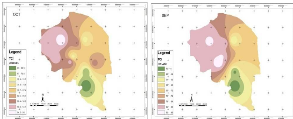
شکل (۸). توزیع زمانی - مکانی اقلیم آسایش گردشگری استان در ماههای سپتامبر و اکتبر
