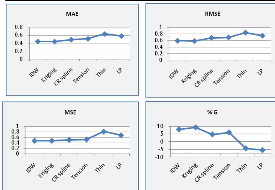
شکل (۳). مقایسه میزان خطا و دقت روشهای مختلف در درون یابی
