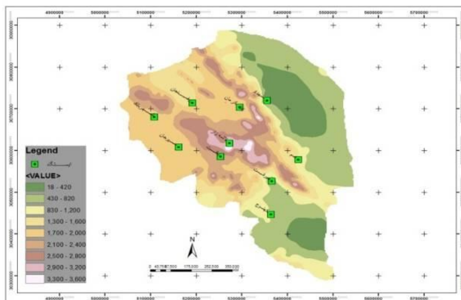
شکل (۲). پراکنش ایستگاه های هواشناسی بر روی نقشه پستی و بلندی منطقه
