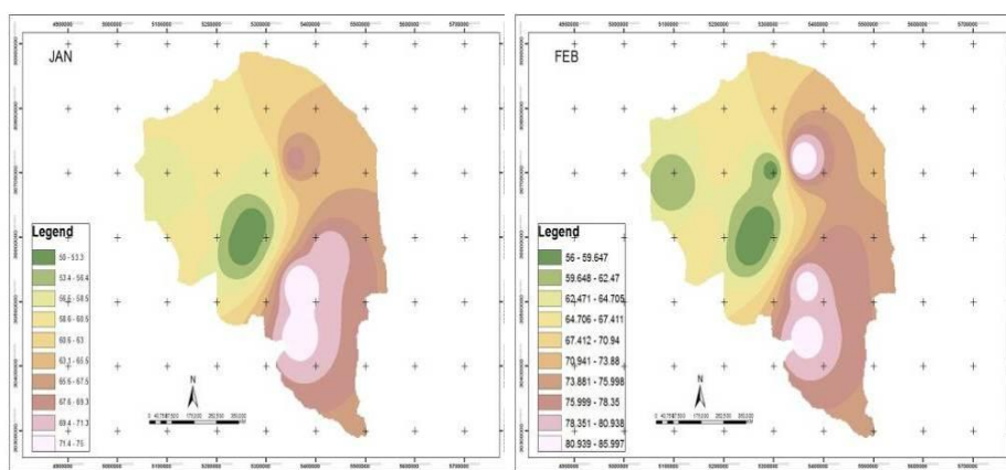
شکل (۴). توزیع زمانی - مکانی اقلیم آسایش گردشگری استان در ماههای ژانویه و فوریه
