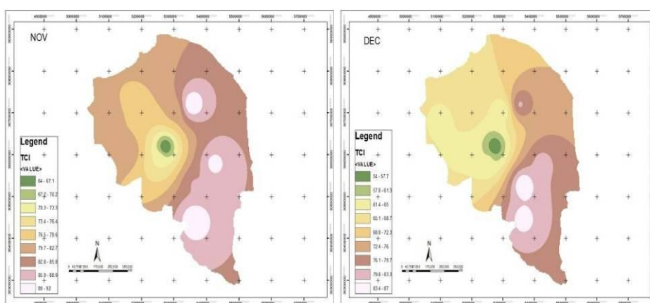
شکل (۹). توزیع زمانی - مکانی اقلیم آسایش استان در ماههای نوامبر و دسامبر
