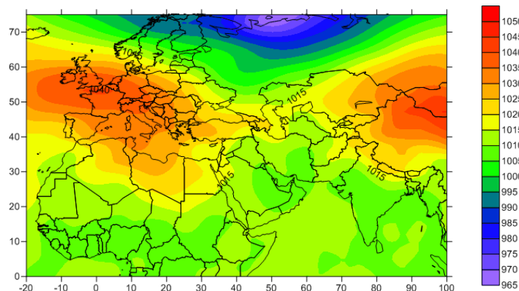
شکل (۹) فشار تراز دریا در روز نماینده الگوی ششم (روز ۱۳۹۰/۱/۳)
