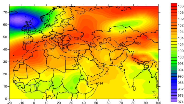
شکل (۸) فشار تراز در روز نماینده الگوی پنجم (روز ۱۳۶۹/۱۲/۲۸)
