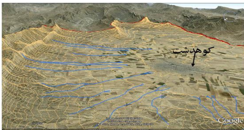
شکل (۱۸) توزیع آبراهه‌های دوشاخه و خطوط تراز بر روی تصویر Google earth دشت کوهدشت
