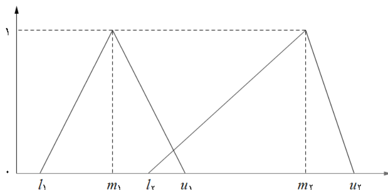
شکل (۲) اعداد مثلثی M_1 و M_2
