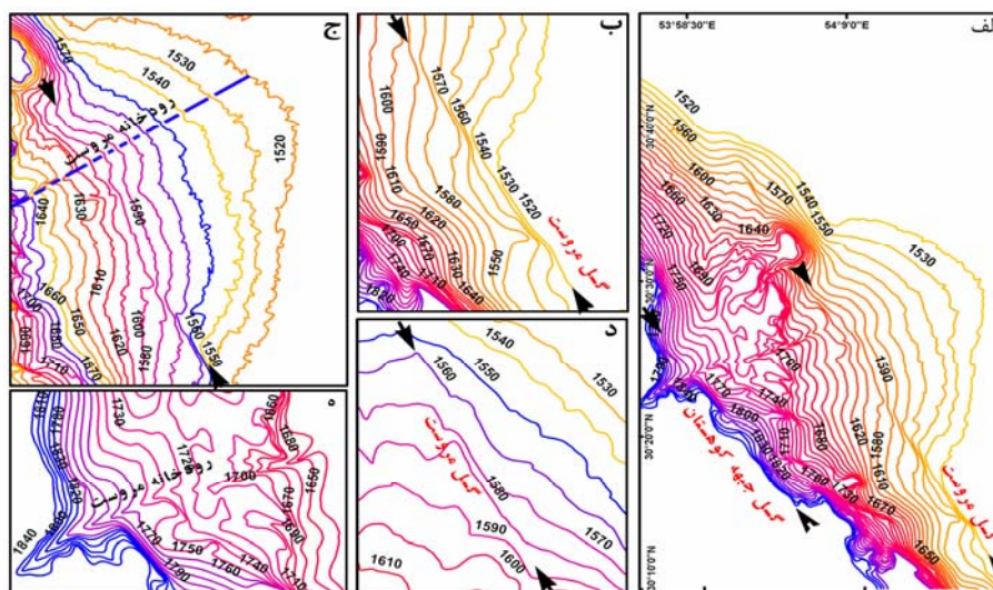
شکل (۹) آشکارسازی تاثیر نوزمینساخت به کمک الگوی منحنی‌های تراز در مخروط‌افکنه مروست
