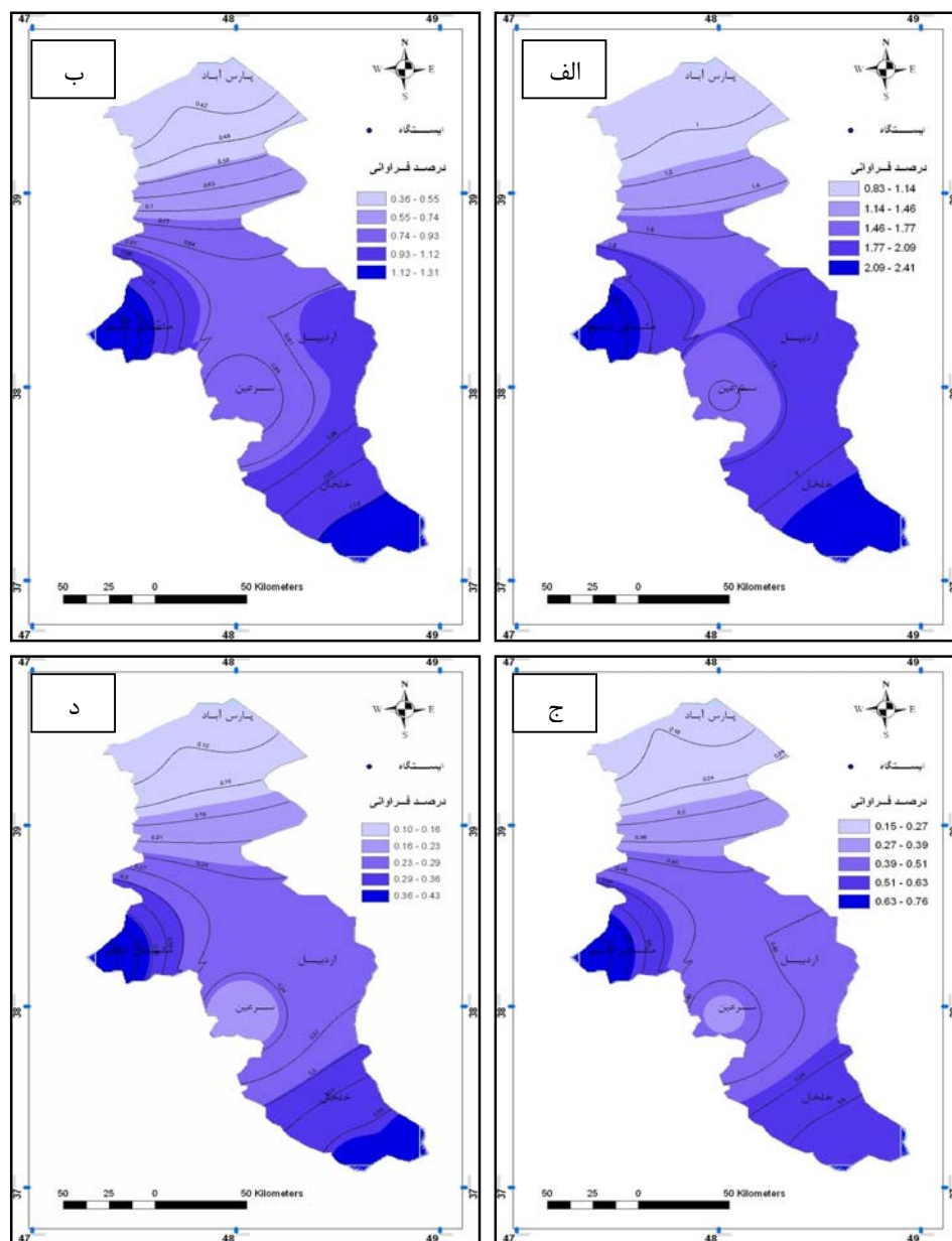
شکل (۶) الف نقشه های هم درصد فراوانی دوره ترزستان (الف) ۴ روزه (ب) ۵ روزه (ج) ۶ روزه (د) ۷ روزه
