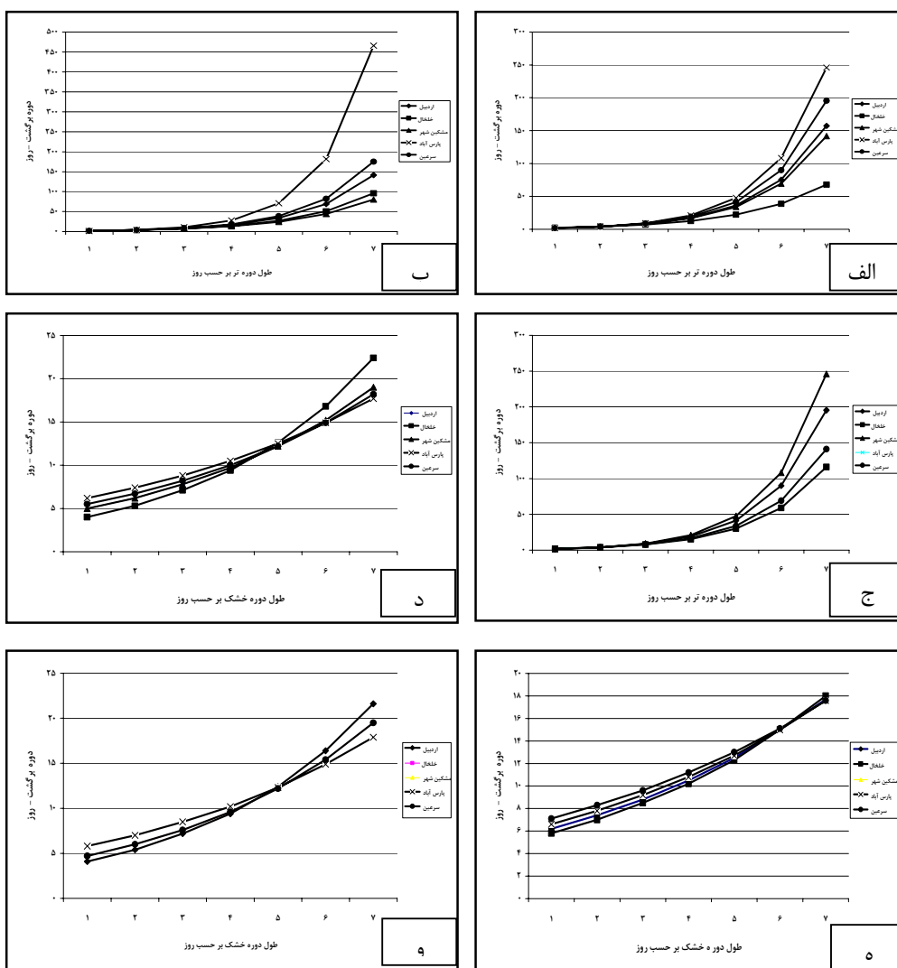
شکل (۴) نمودار دوره های برگشت موسم های تر (الف) زمستان (ب) بهار (ج) پاییز و دوره های برگشت موسم های خشک (د) زمستان (ه) بهار (و) پاییز
