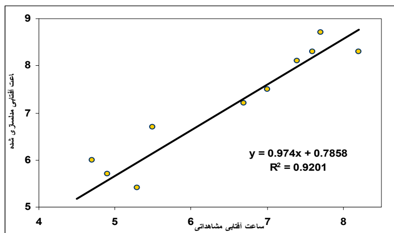
شکل (۶) الف و ب: نمودار پراکنش ساعت آفتابی و بارش ماهانه مشاهداتی و مدل سازی شده گرگان (۱۹۹۳-۲۰۰۷)
