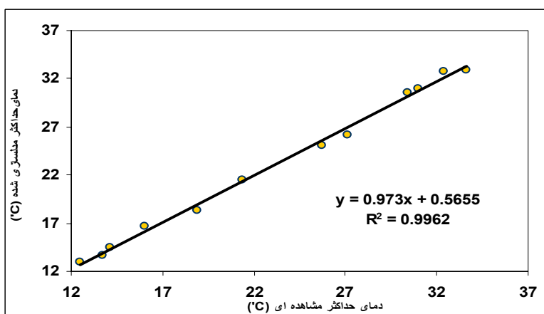
شکل (۵) الف و ب: نمودار پراکنش دمای حداکثر و حداقل ماهانه مشاهداتی و مدلسازی شده گرگان (۱۹۹۳-۲۰۰۷)
