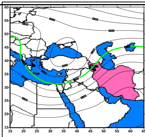
الگوی دوم (سردچال بالایی شمال ترکیه)
