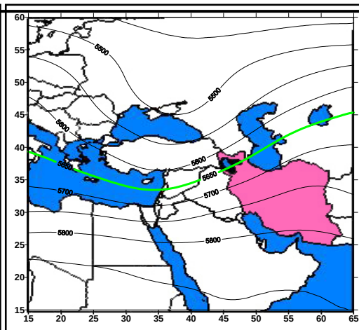
الگوی اول (تراف موج کوتاه دریای سیاه)
