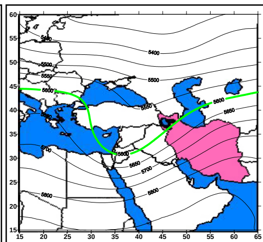
الگوی سوم (تراف موج کوتاه سواحل شرق دریای مدیترانه) الگوی چهارم (سردچال بالایی شمال دریای سیاه)
