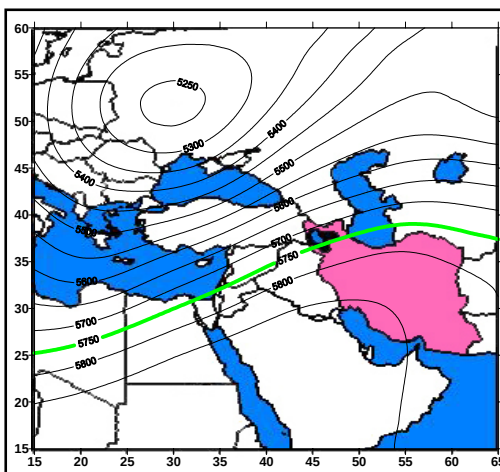
الگوی سوم (تراف موج کوتاه سواحل شرق دریای مدیترانه) الگوی چهارم (سردچال بالایی شمال دریای سیاه)
