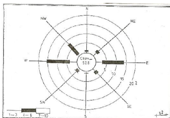
شکل ۸. وضعیت گلباد سالانه ایستگاه سینوپیتیک قم.
