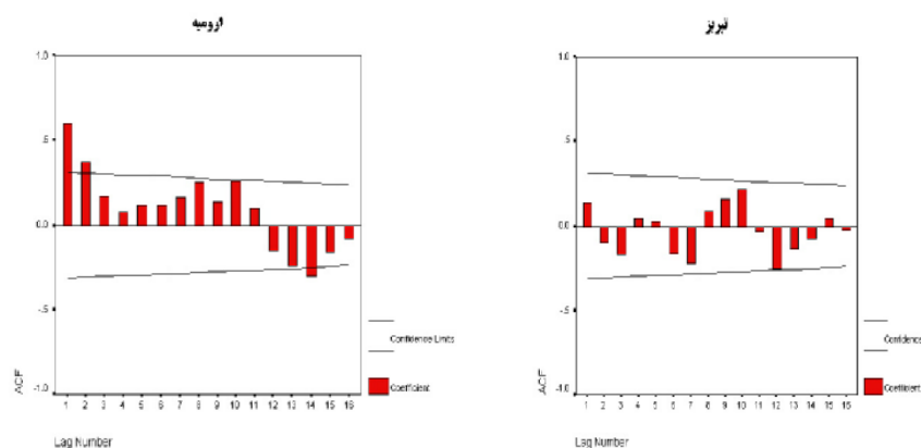
شکل ۲: رفتار تابع خود همبستگی داده‌های دمای متوسط ایستگاه تبریز و ارومیه
