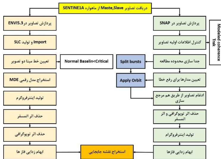
شکل (۵). فلوچارت مراحل پردازش در نرم افزار SNAP و SARscape
