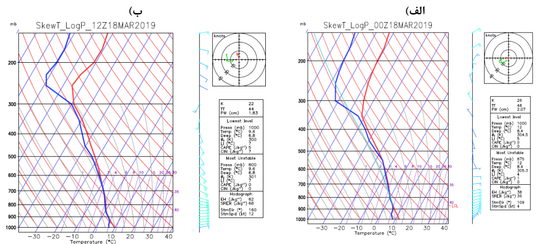
شکل (۸). الف) نمودارهای ترمودینامیکی ساعت ۰۰۰۰ وب ۱۲۰۰ گرینویچ روز ۲۷ اسفند ۱۳۹۷ ایستگاه گرگان
